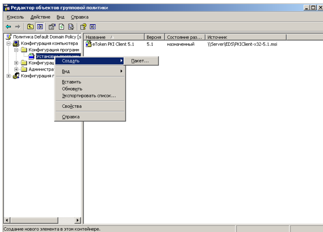
Рис. 1.3.5 – Добавление дистрибутива в список устанавливаемых программ
